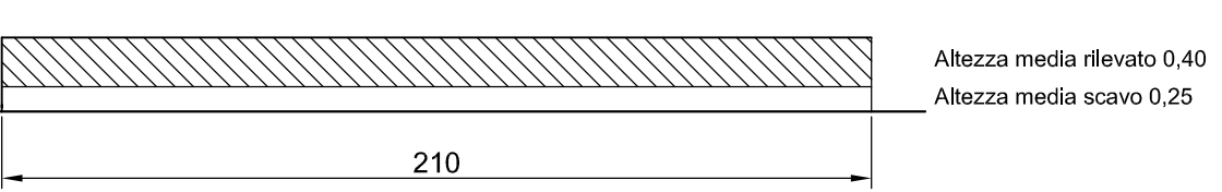
Sezione schematica rilevato c-c'
